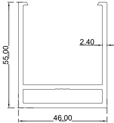
عمود باب خارجي مع غطاء (55*46) ملم الرقم التسلسلي للصنف: BLT4009 الوزن: 1.270:(Kg/m)
