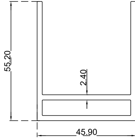
عمود باب خارجي بدون غطاء (45.9*55.2) ملم الرقم التسلسلي للصنف: BLT1952 الوزن: 1.257:(Kg/m)
