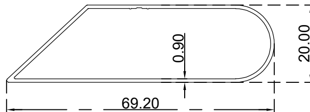
معيّن (20*69.2)ملم الرقم التسلسلي للصنف: AS00001 الوزن 0.379:(Kg/m)
