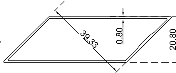
معيّن (20*40)ملم الرقم التسلسلي للصنف: BLT3285 الوزن 0.376:(Kg/m)
