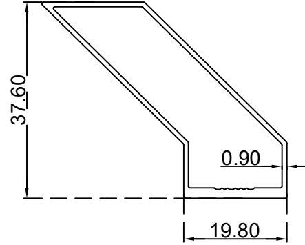
رفراف زاوية 45 الرقم التسلسلي للصنف: BLT1954 الوزن 0.377:(Kg/m)
