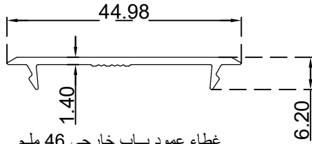
غطاء عمود باب خارجي 46 ملم الرقم التسلسلي للصنف: BLT4010 الوزن 0.202:(Kg/m)
