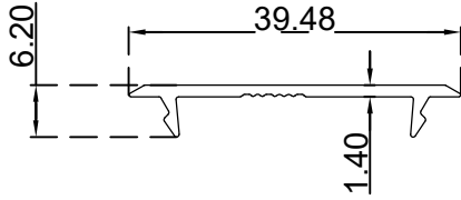
غطاء عمود باب خارجي 40.5 ملم الرقم التسلسلي للصنف: BLT4368 الوزن 0.173:(Kg/m)
