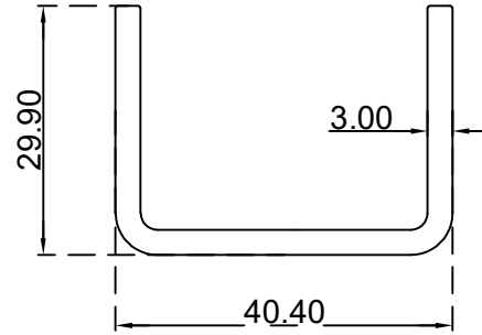
عمود باب خارجي يو (29.9*40.4) ملم الرقم التسلسلي للصنف: C40.4*29.9*3.0 الوزن: 0.744:(Kg/m)
