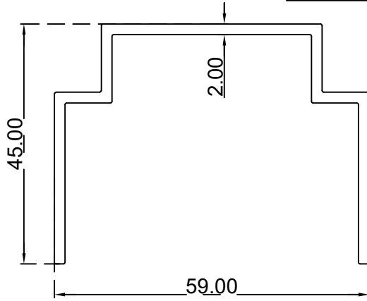
عمود باب خارجي يو (45*59) ملم الرقم التسلسلي للصنف: BLT1953 الوزن: 0.788:(Kg/m)
