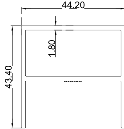
عمود باب خارجي بدون غطاء (44.2*43.4) ملم الرقم التسلسلي للصنف: BLT3605 الوزن: 0.849:(Kg/m)
